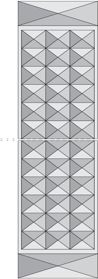
Spalla Cuspidi Classica Spessore 7,5 Cm Side Classic Cuspide th. 7,5 cm
