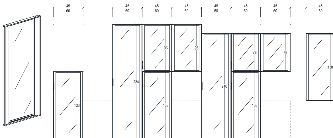
Finitura karbon (vedi sezione Brera) Karbon finish (see Brera section)
